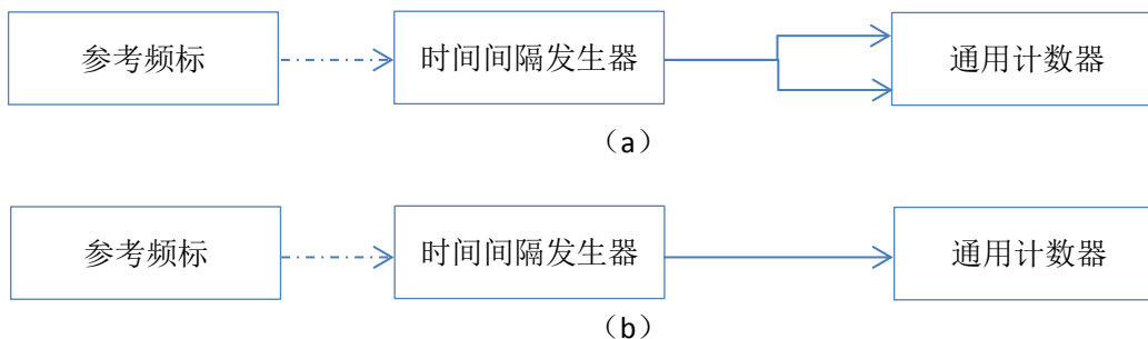
正、负脉冲宽度测量误差检定框图
